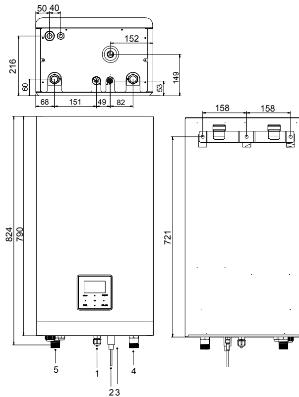
Afb. 4-2 eenheid: mm
